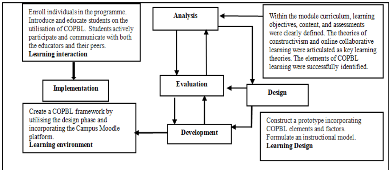
Fig 1. COPBL framework
