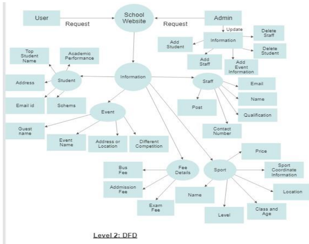
Fig 1 DFD
