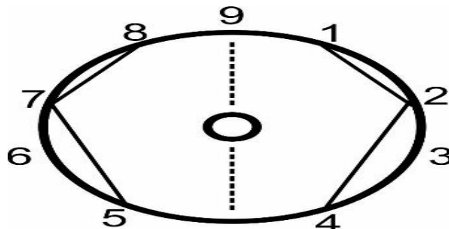
Fig. 2: EOF
