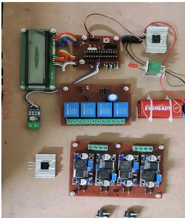
Fig 1:- Module
